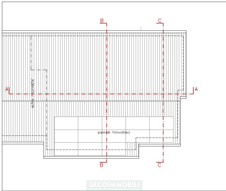
PIANTA COPERTURA
