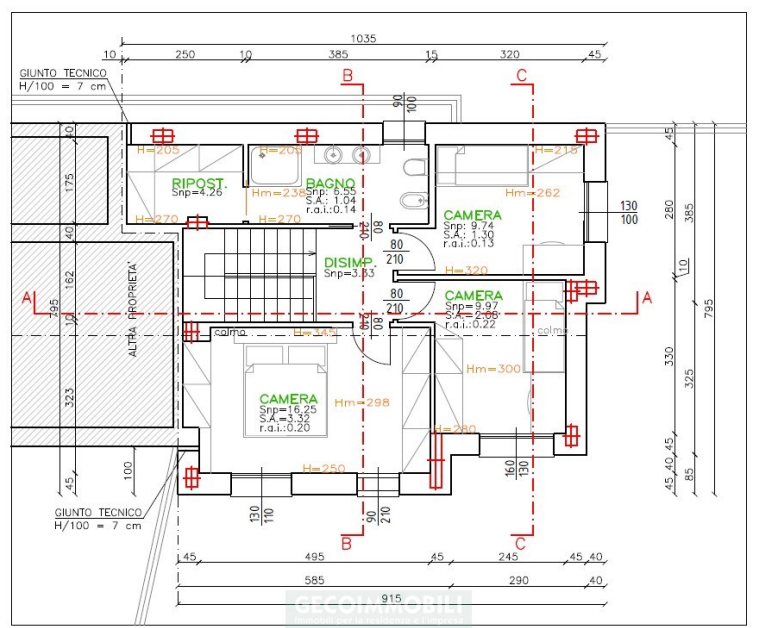
PIANO PRIMO
