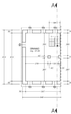
PIANTA SOTTOTETTO
