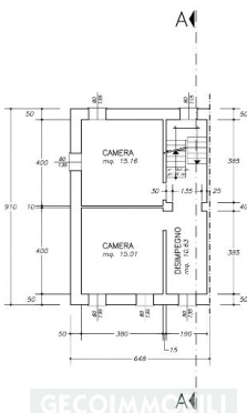
PIANTA PRIMO PIANO
