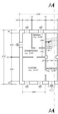
PIANTA PIANO TERRA
