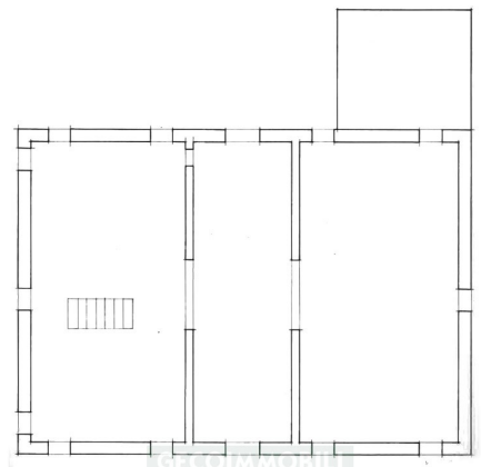
PIANO SOTTOTETTO
