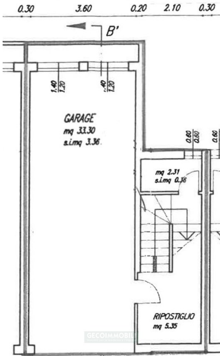
PIANTA PIANO INTERRATO
