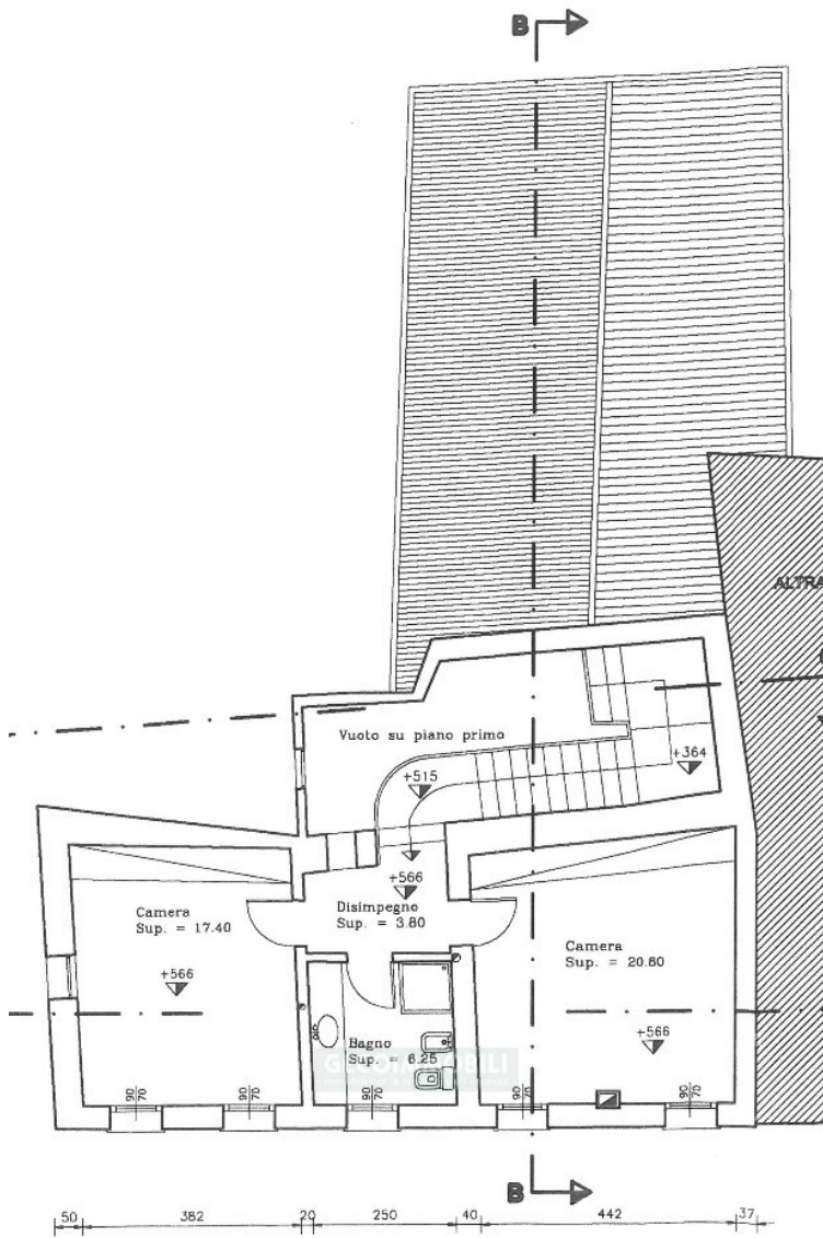
PIANO SECONDO
