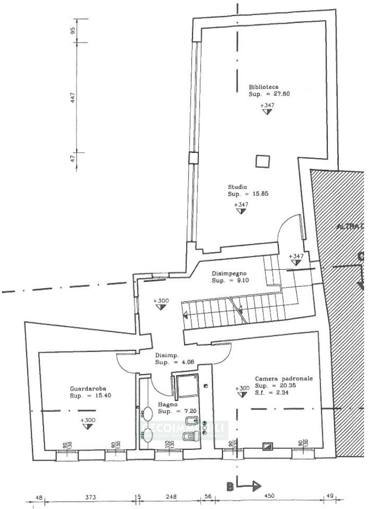
PIANO PRIMO
