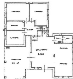
PIANTA PIANO TERRA H. 270
