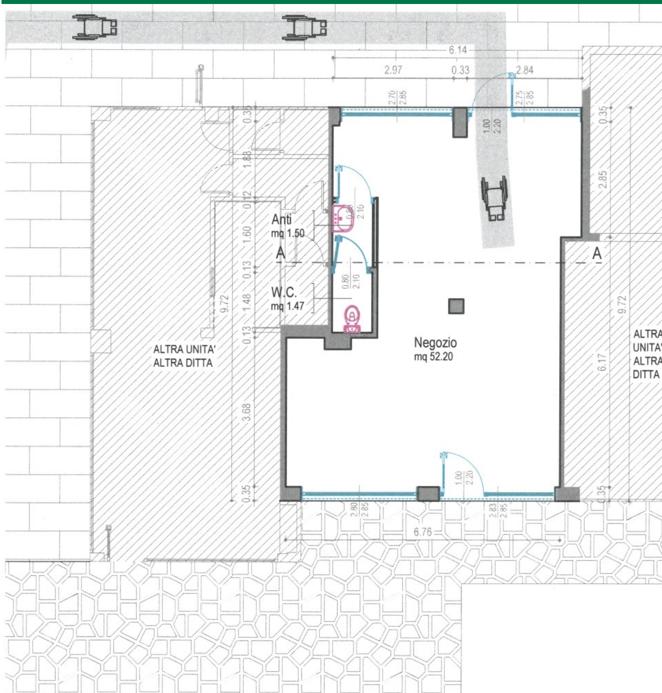
PIANTA PIANO TERRA - PROGETTO
