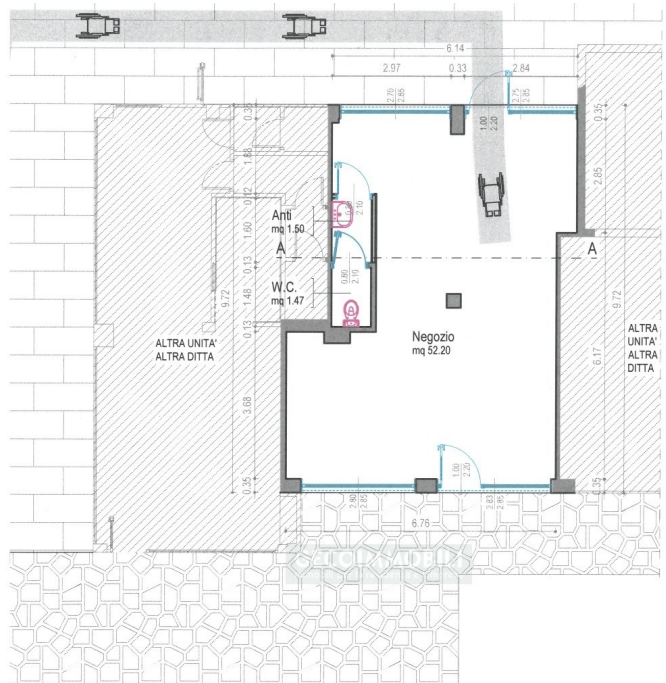
PIANTA PIANO TERRA - PROGETTO
