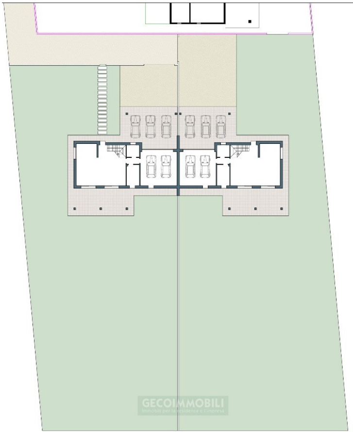
PLANIMETRIA STATO DI PROGETTO, scala 1:200
