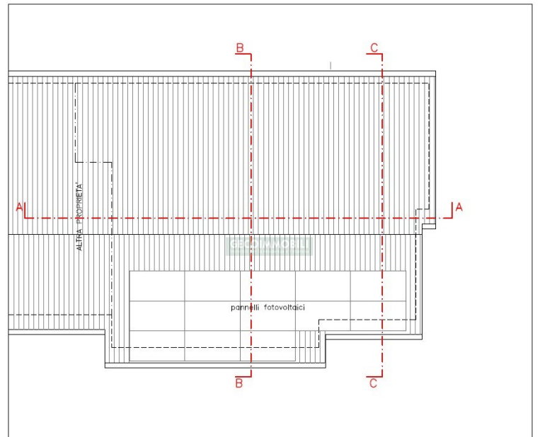
PIANTA COPERTURA
