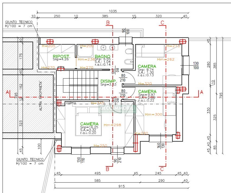
PIANO PRIMO
