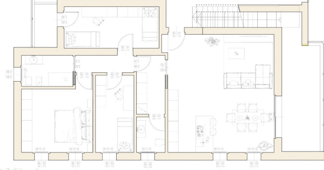
PIANO PRIMO
